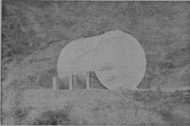
Tanque metálico de almacenamiento, colocado horizontalmente, del acueducto de Tempate de Santa Cruz. Este depósito de agua tiene 25.000 litros de capacidad.
