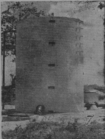
Tanque metálico de almacenamiento del acueducto de San Roque de Liberia, con capacidad de 25.000 litros.
